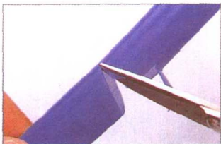
9、将多余修剪(欲折弯处)
