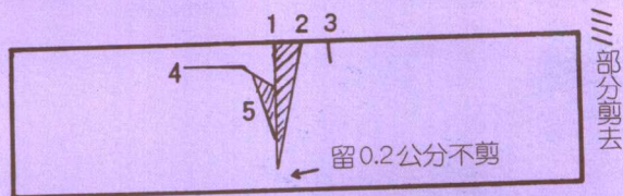
1、垂直剪圆管,留约0.2公分不要剪断。
