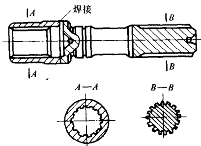
图 0-1 拖拉机半轴
