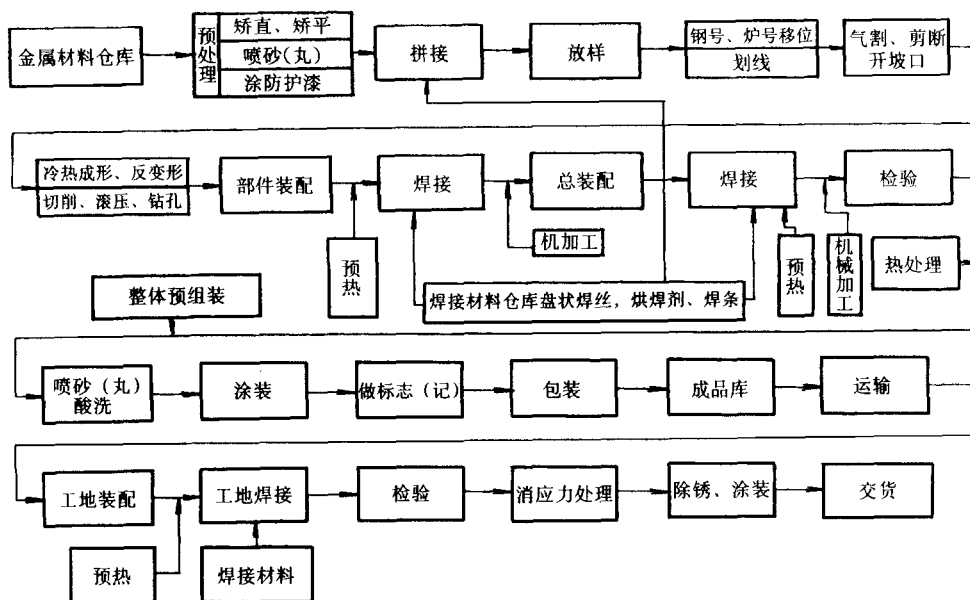
图 0-5 一般焊接结构生产的主要工艺过程
