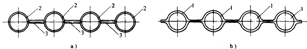
图 0-3 型材与焊接结构的比较
