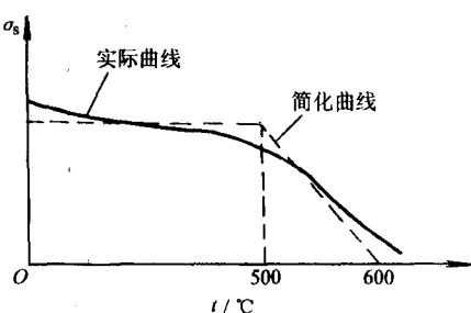
图 1-2 低碳钢的屈服点与温度的关系
