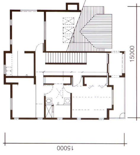
二层平面图
