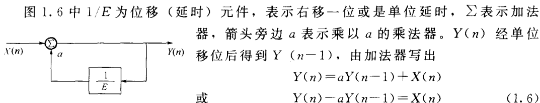
图 1.6 一简单离散系统示意
