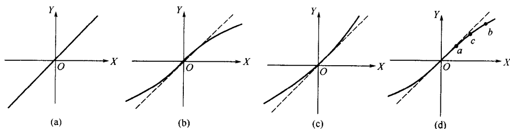
图 1.7 检测系统的四种典型静态特性
