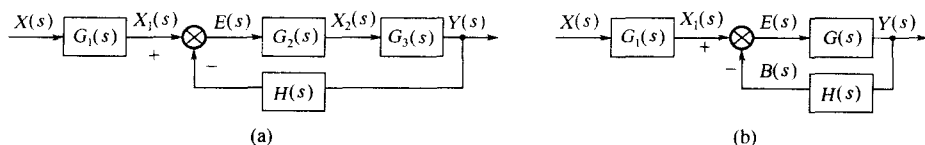
图 1.5 闭环检测系统结构
