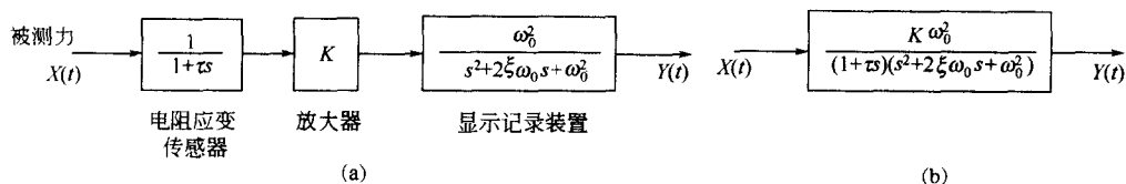
图 1.3 一个应力应变检测系统的传递函数
