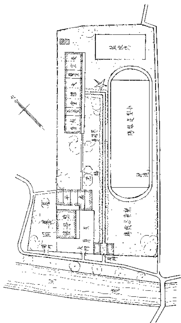
時化小學校舍平面圖
