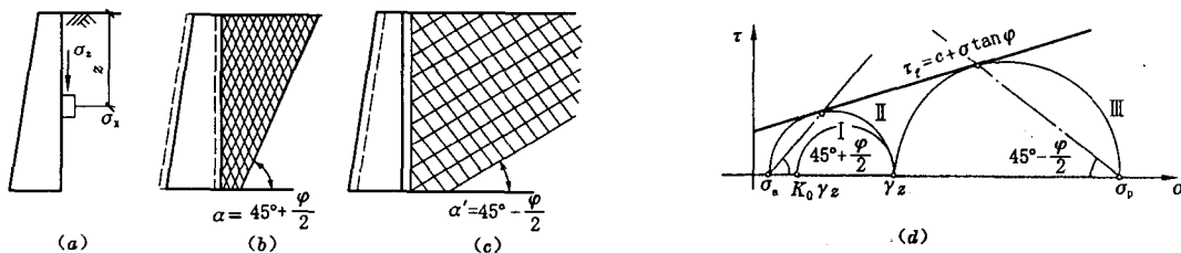
图 2.4 半空间的极限平衡状态
