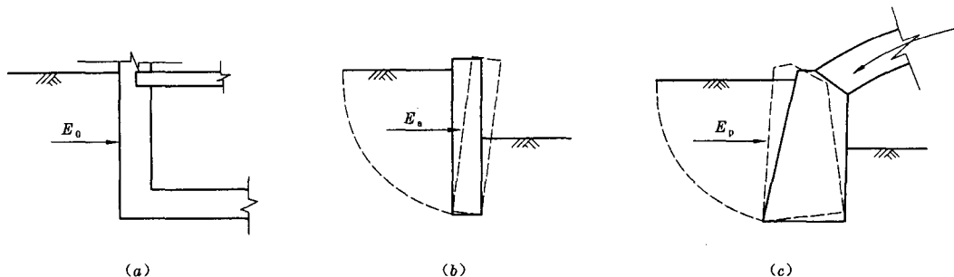
图 2.3 挡土墙的三种土压力
