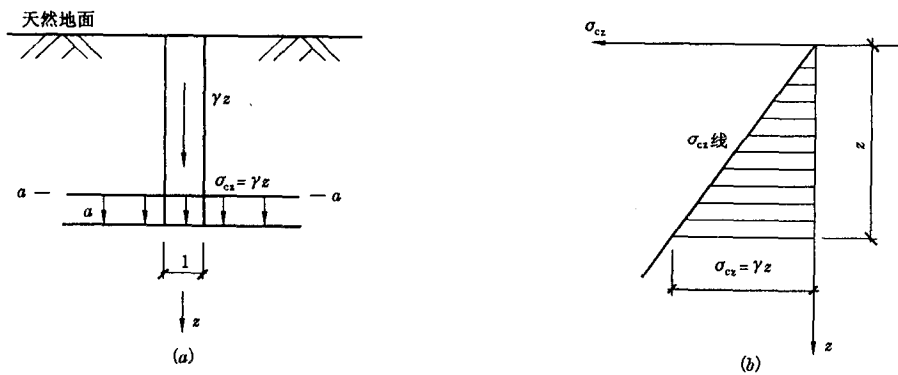
图 2.1 均质土中竖向自重应力
