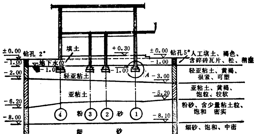
图2-1 建筑物地基基础示意
