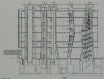
剖面图
