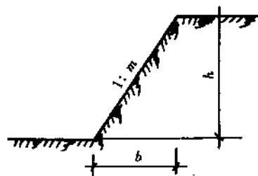
图 1-2 土方边坡
