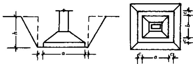
图 1-4 基坑土方量计算
