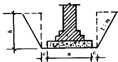
图 1-3 基槽土方量计算
