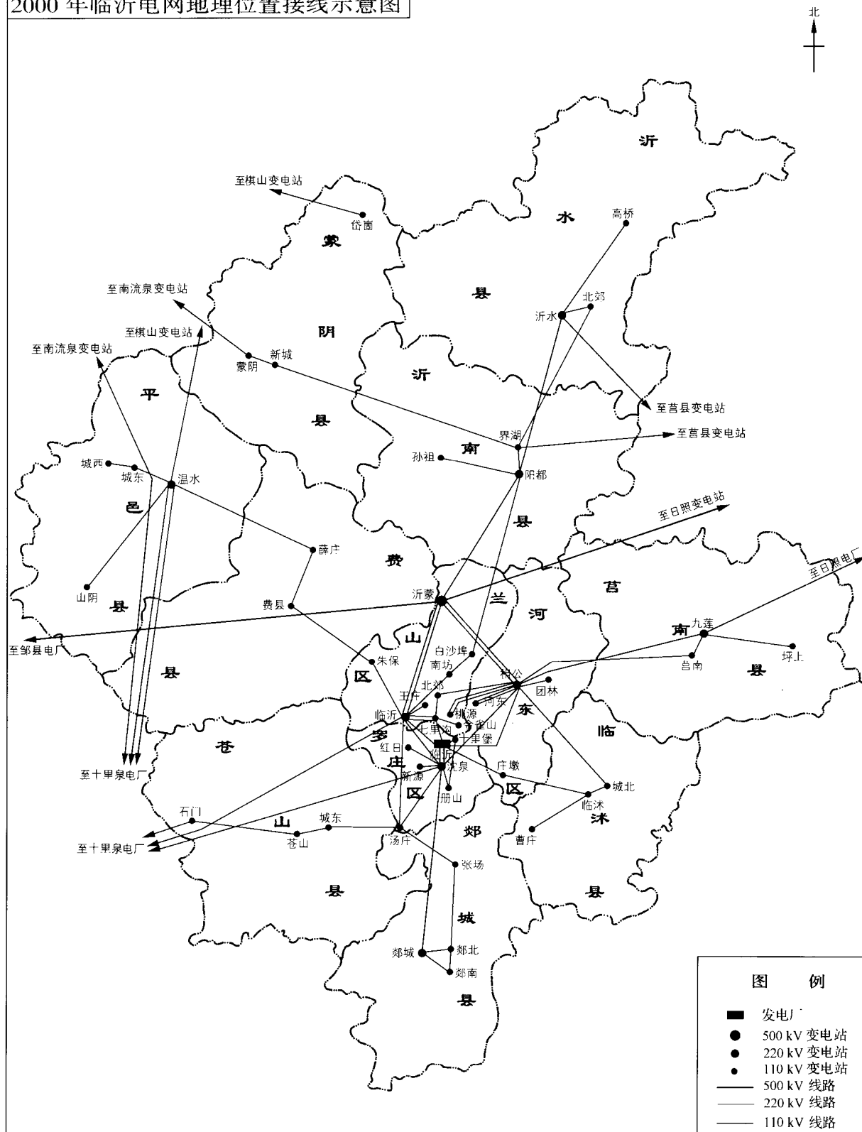
2000 年临沂电网地理位置接线示意图
