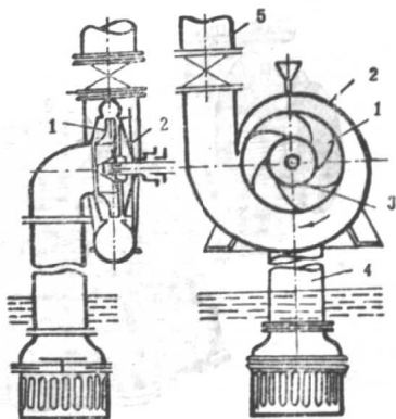
图1—3 离心泵的结构示意图
