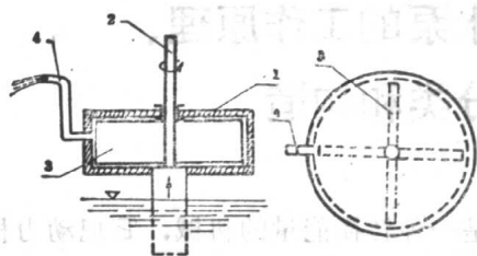
图 1—2 利用离心力抽水示意图
