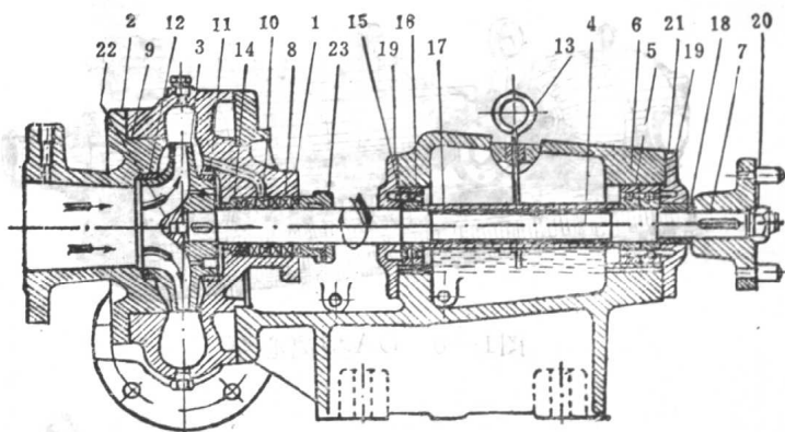
图1—8 乙式BA型离心泵的构造
