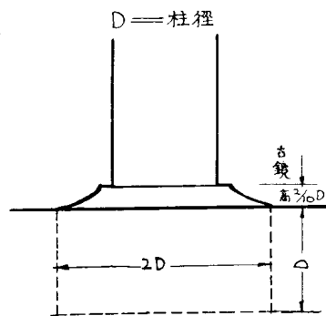
上圖按宋營造法式卷五繪
