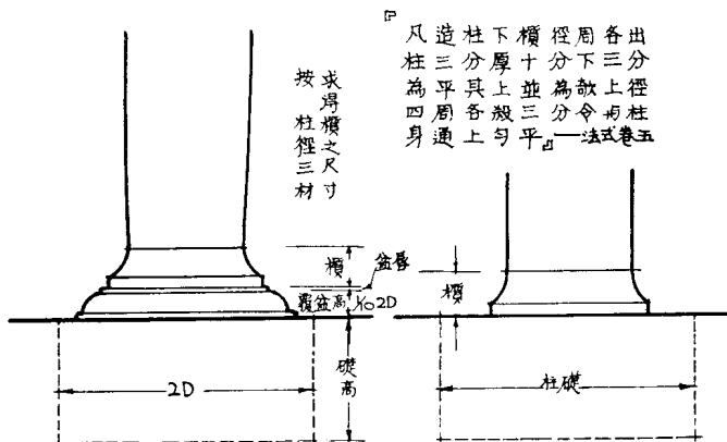
上圖按宋營造法式卷五繪
