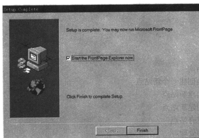
图 1.12 安装完成
