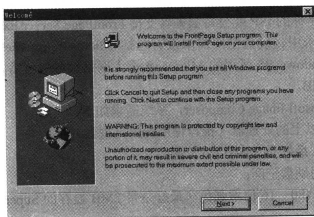
图 1.2 欢迎画面
