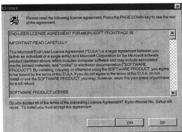
图 1.6 授权对话框
