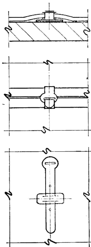
粘接法鋁皮軌安裝圖 (排線寬度 \leq 20\text{mm} )
