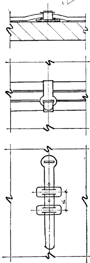
粘接法鋁皮軌安裝圖 (排線寬度 \geq 20\text{mm} , \leq 30\text{mm} )
