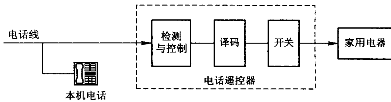
图 1-2 电话遥控器的组成
