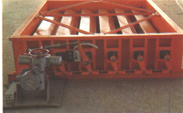
青岛电站辅机厂生产的“辉煌”牌 GBM型(S0—600mw)电站风门 (获 1990 年国家质量银质奖)
