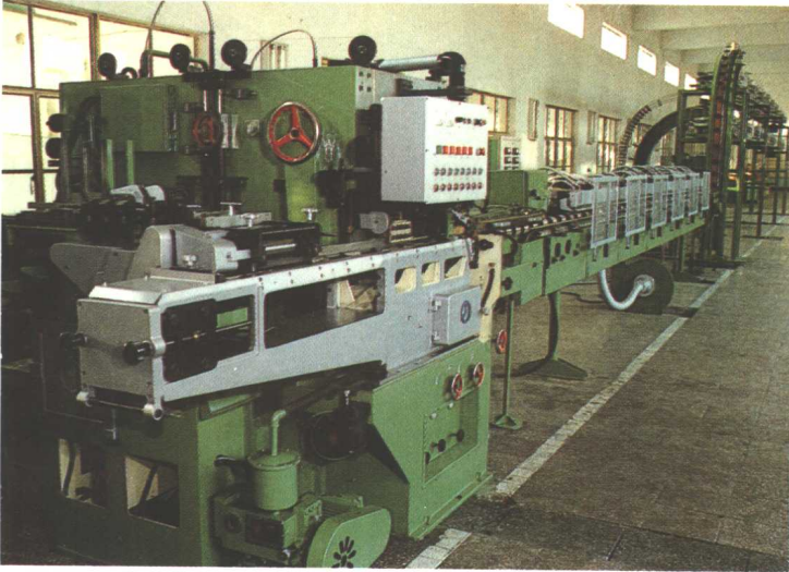
青岛锻压机械厂生产的电阻焊三片罐自动生产线 (获中国首届食品博览会金奖和机械部科技进步一等奖)。
