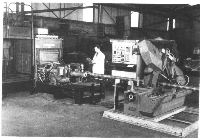
RT850 型连铸机，带移动自动带锯切断装置
