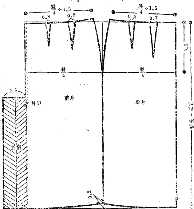
暗裥裙裁剪制图
