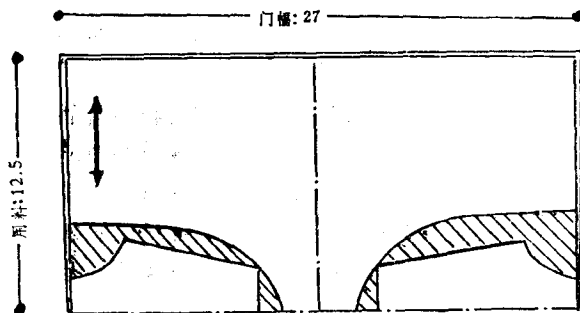
排料图之二、对折排料
