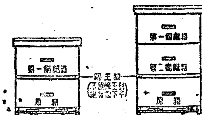
圖9 繼箱
