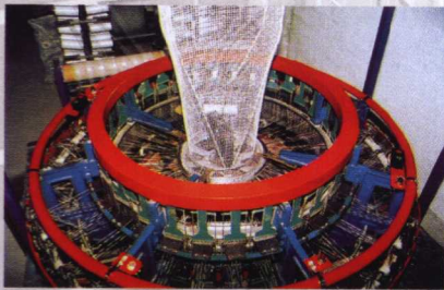
四梭网眼圆织机 Four-shuttle Network Circular Loom
