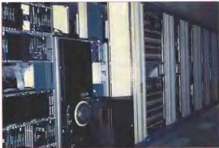
程序控制数字电话交换机一角
