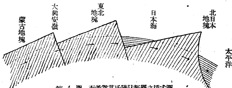
第4圖 李希霍芬氏階狀斷層之模式圖
