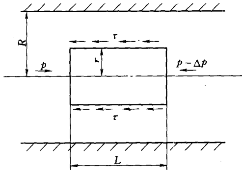
图 1.4 圆形导管中流动液体受力分析
