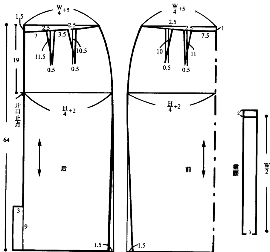
图 2-7 裙子裁剪图
