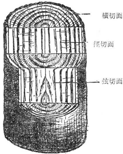
圖1 木材的三個切面
