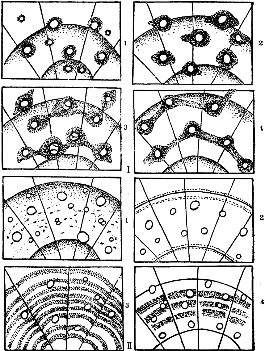
圖 4 木薄壁組織排列的類型
