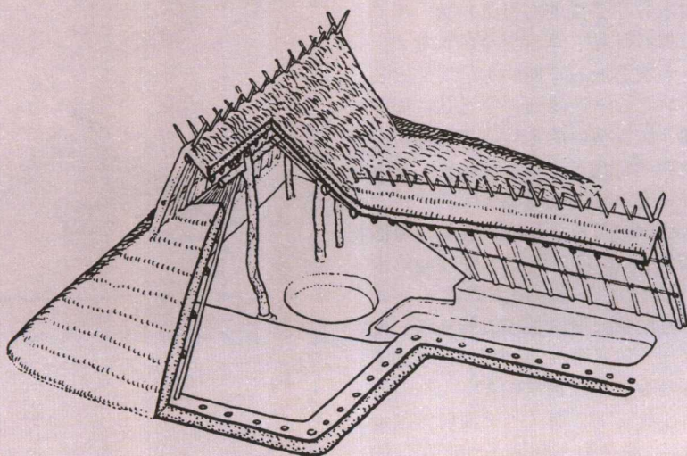
剖视 (复原想像)
