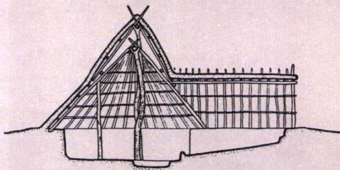
剖面 I—I (复原想像)
