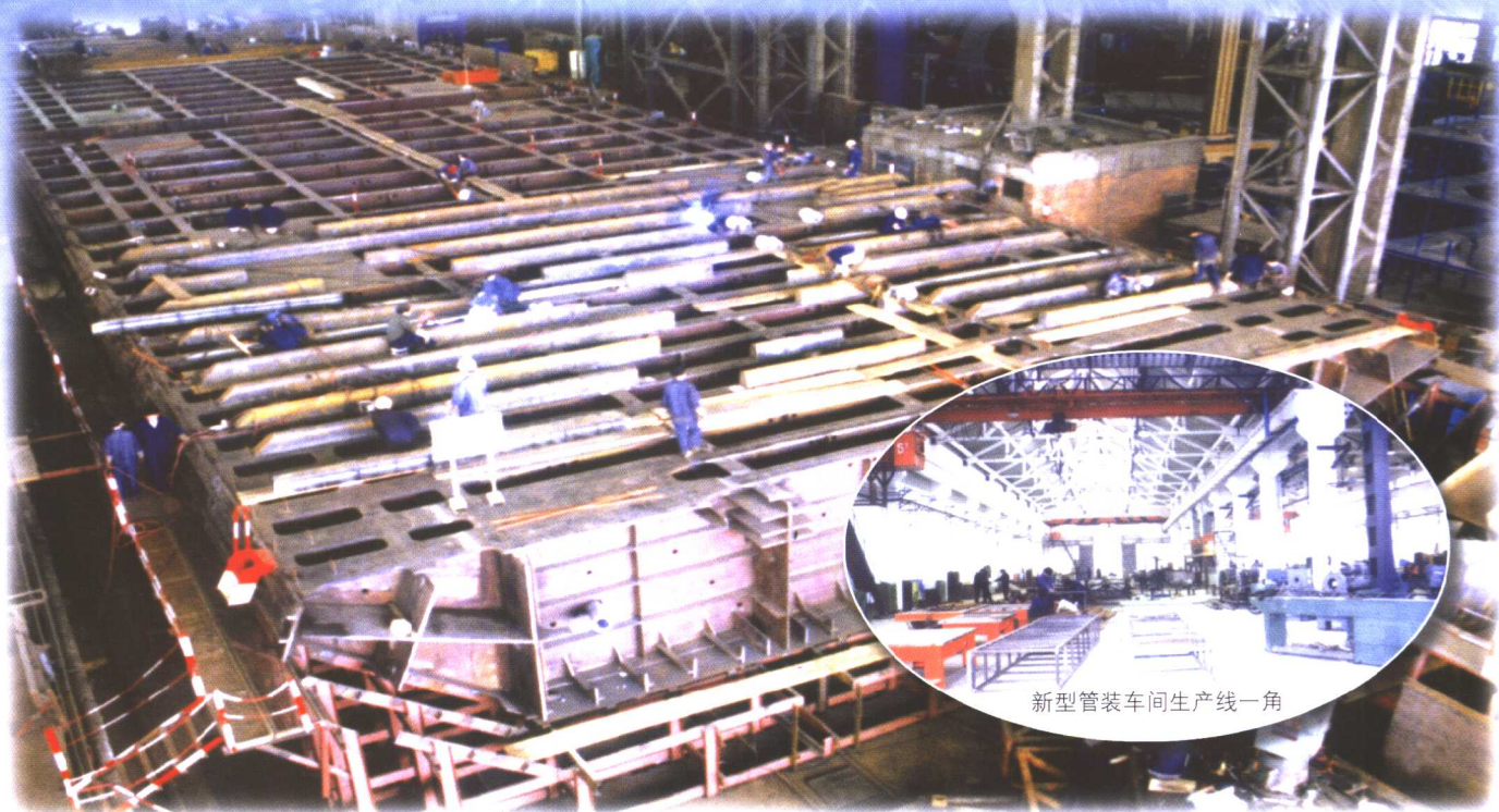
三峡永久船闸厂内施工
