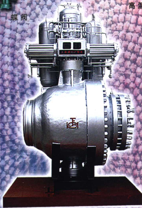
DN1000mm PN8MPa 大球阀
