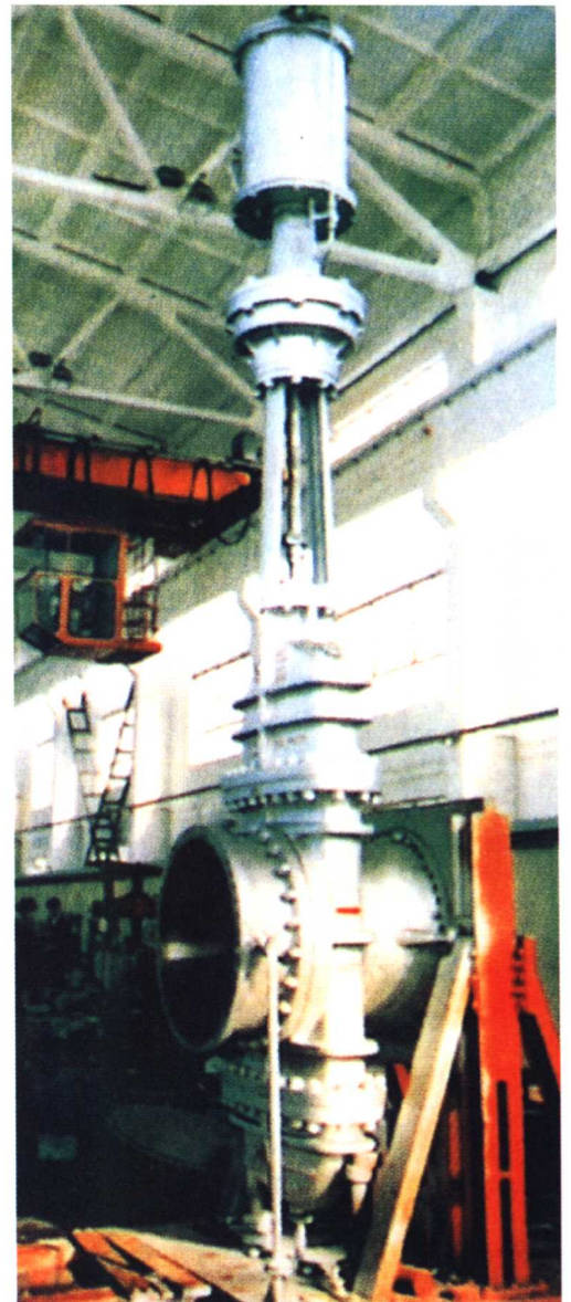
32" 气动平板闸阀
