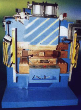
微波炉波导管专用焊机 PW-C30000J
