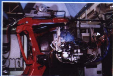
机器人弧焊系统
