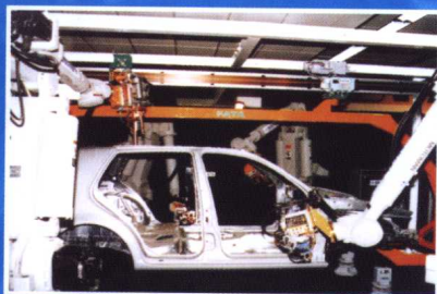
机器人点焊系统
