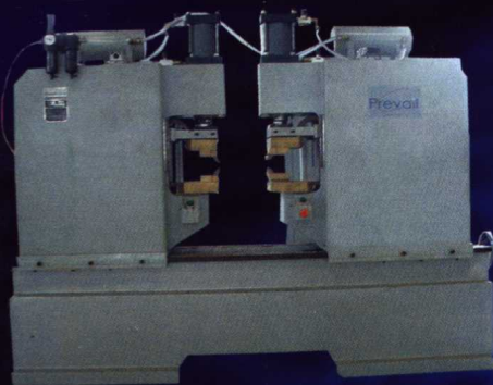
微波炉腔体自动焊接专机 PW-CD9000J
