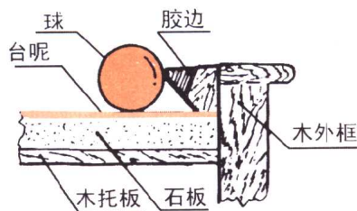
图 1-6 球台剖面图
