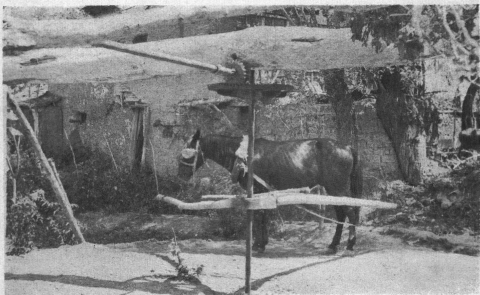
土耳其鄉村中,老式的輪磨機係用馬力。
