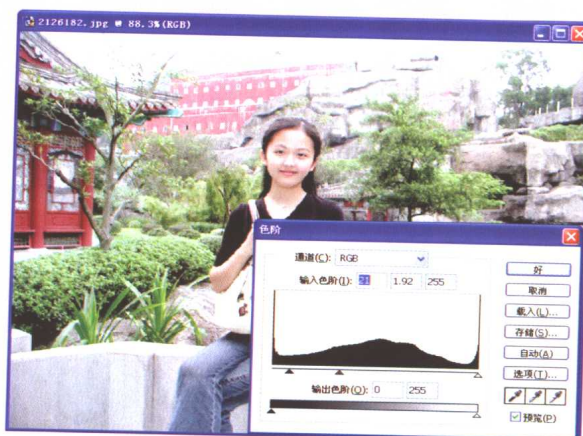
图 5-110 【色阶】对话框
