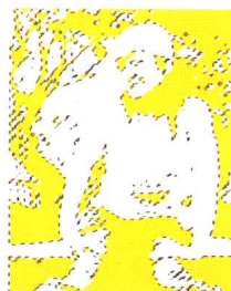
图 5-339 填充效果(2)
