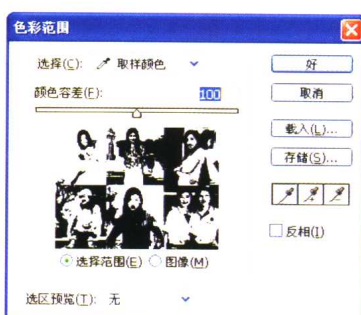
图 5-334 色彩范围
