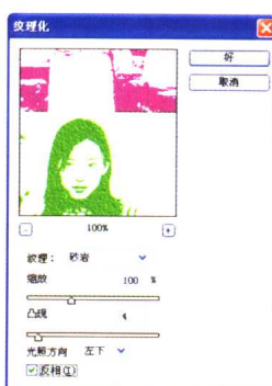
图 5-346 纹理化
