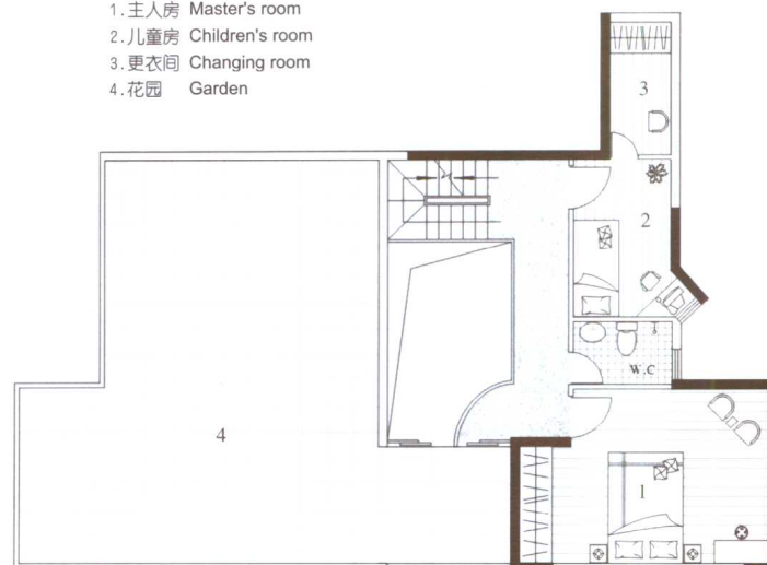
二层平面图 2F plan view
