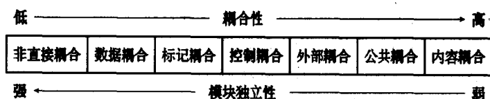
图 1-2 模块之间的耦合性
