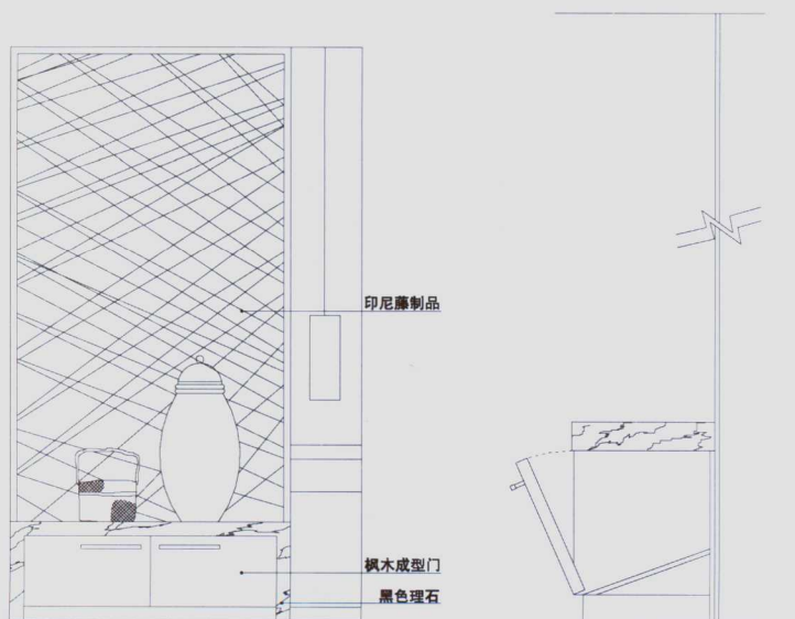
重要节点图
