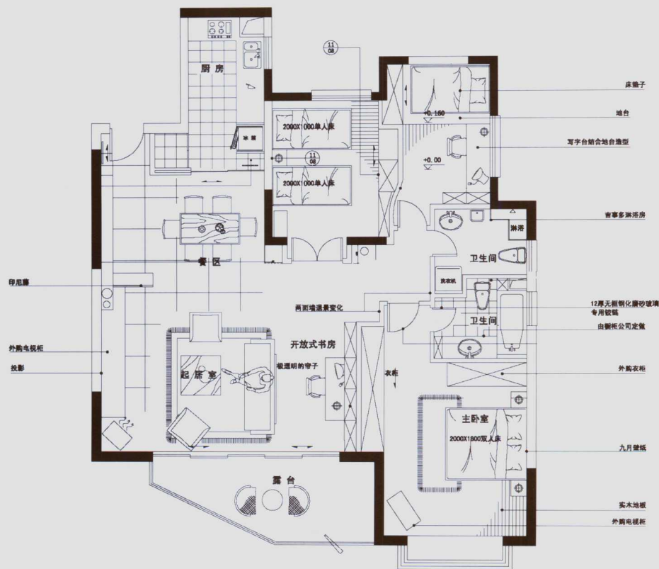
平面布置图
