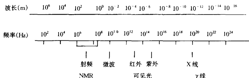
线图 1-1-1 电磁波谱
