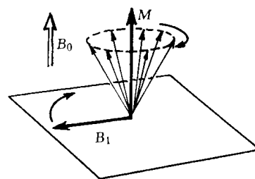
线图 1-2-1 射频脉冲效应示意图
