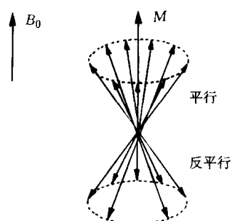
线图 1-1-7 某一瞬间的大量自旋模型
