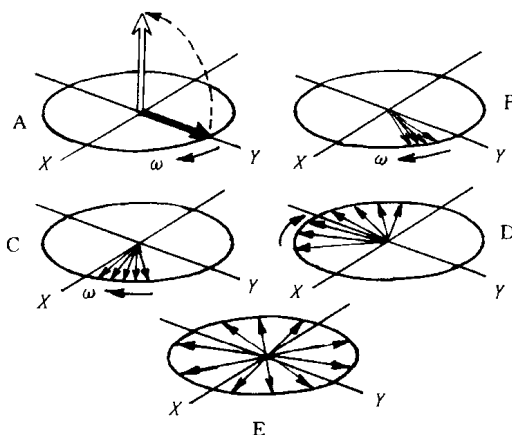
线图 1-2-5 横向磁化矢量相位离散
