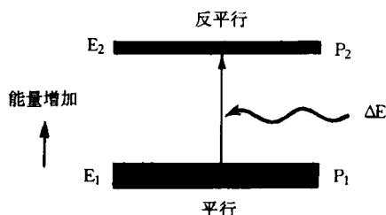
线图 1-1-5 核自旋择优取向后的能态示意图
