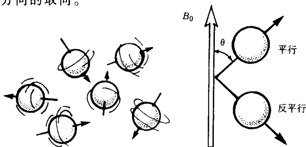
线图 1-1-3 无外磁场时核磁矩排列示意图
