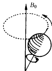
线图 1-1-6 核自旋拉摩进动
