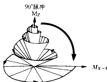
线图 1-2-2 磁化矢量的螺旋倾倒方式
