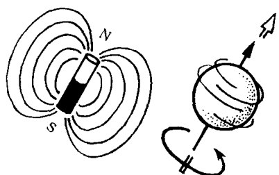
线图 1-1-2 核自旋示意图
