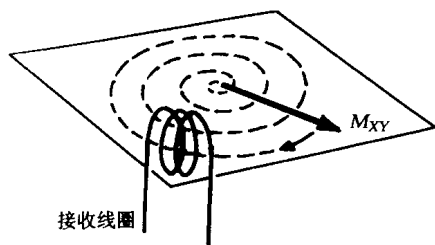
线图 1-2-3 自由感应衰减(FID)形成示意图 横向磁化矢量绕着主磁场 B_0 以拉摩频率进动。旋转的磁化矢量会在接收线圈内感应一交变电流。
