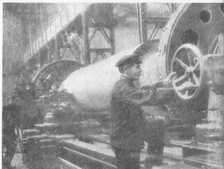
↑ (45)兩個五年計劃使蘇聯成為經濟上獨立的國家，蘇聯已學會了用自己的力量設計和修建任何種類的工廠，沒有一種機器是蘇聯所不能製造的。圖為依若爾機器製造廠的一架巨型車床在車製鋼板軋壓機的滾軸。
