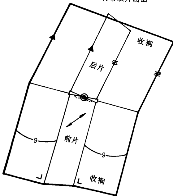
背带展开制图
