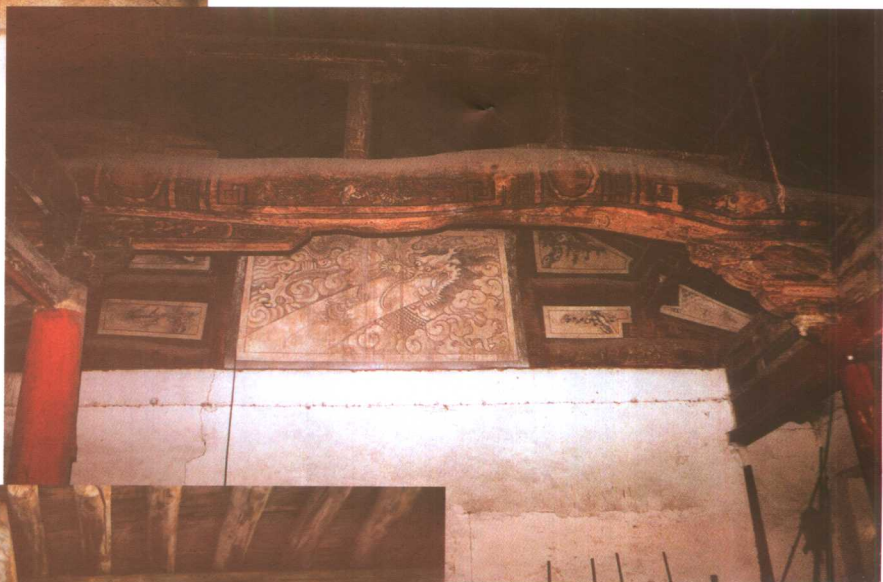
襄垣大成殿内部梁架
