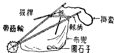
第三圖 粘虫車
