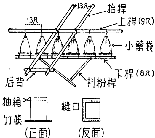
第一圖 轆式布袋撒粉器
