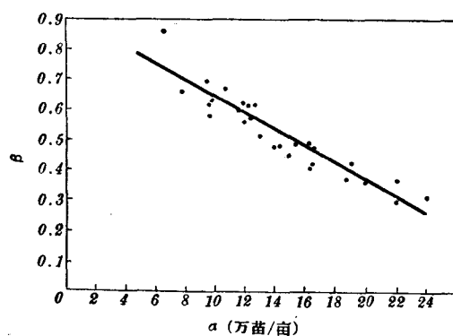
图5 基本苗数与有效穗数的回归直线( y_w = \alpha + \beta y_0 )中 \alpha 及 \beta 的相关图
