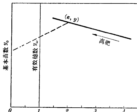
图 6 基本苗数与有效穗数 相互推算用的列线图
