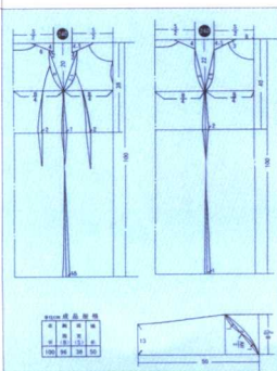
裁剪图 63 - 125
