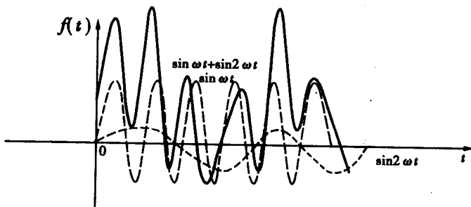
图 1.1-7 合成信号是一个非正弦周期信号
