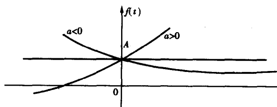
图 1.1-9 连续时间实指数信号
