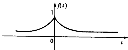
(a) f_1(t) = e^{-2|t|}
