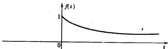
图 1.1-4 非功率能量信号
