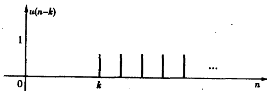
图 1.1-18 离散时间单位阶跃序列
