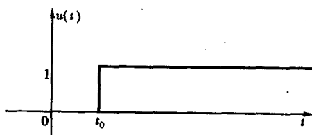
图 1.1-15 延迟连续时间单位阶跃信号
