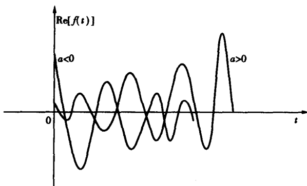
图 1.1-12 复指数信号的实部是一个增幅( a > 0 )或减幅( a < 0 )的余弦信号
