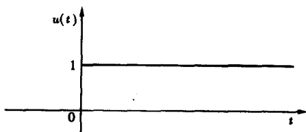
图 1.1-14 连续时间单位阶跃信号
