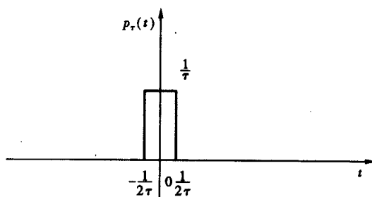
(b) 连续时间信号矩形脉冲 p_\tau(t)
