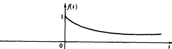
图 1.1-1 连续时间信号
