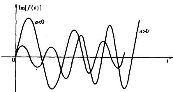
图 1.1-13 复指数信号的虚部是一个增幅( a > 0 )或减幅( a < 0 )的正弦信号
