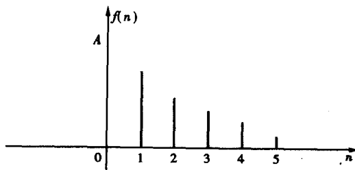
图 1.1-2 离散时间信号
