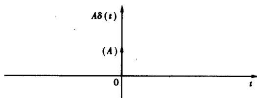
图 1.1-20 连续时间冲激信号
