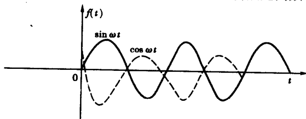
图 1.1-8 正弦信号对时间的微分或积分仍然是同频率的正弦信号
