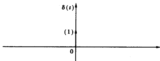
图 1.1-19 连续时间单位冲激信号
