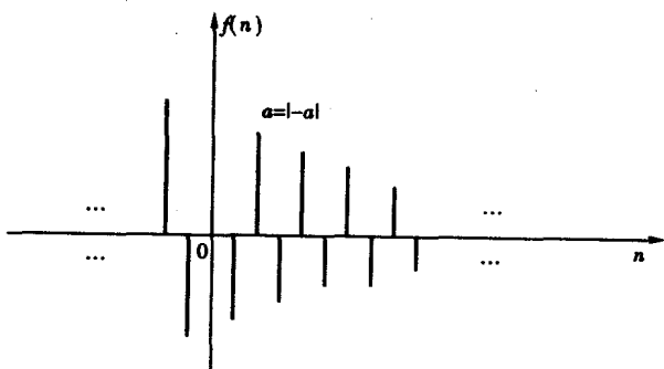
图 1.1-11 在实数 a = |-a| 时的实指数序列
