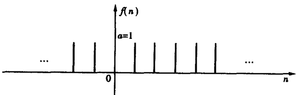
(b) 在实数 a = 1 时的实指数序列
