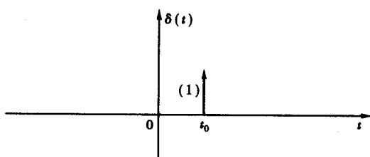
(a) 延迟连续时间单位冲激信号
