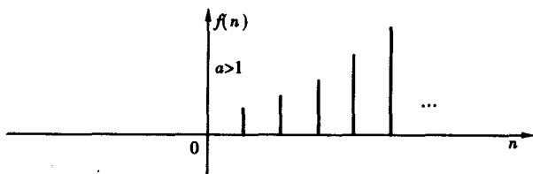
(a) 在实数 a > 1 时的实指数序列
