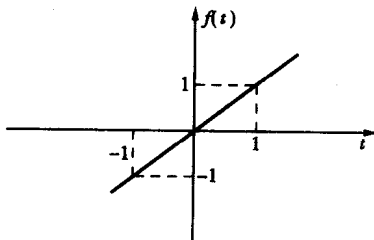
图 1.1-5 非功率非能量信号
