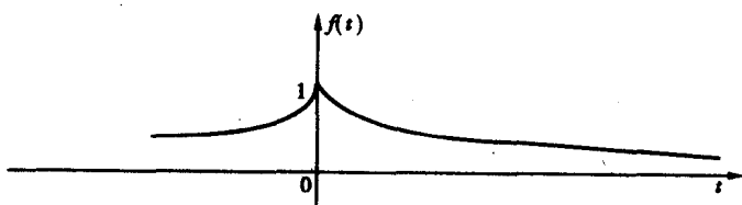
图 1.1-16 连续时间因信号和反因信号
