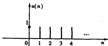
图 1.1-17 离散时间单位阶跃序列
