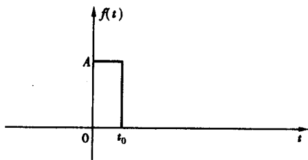
图 1.1-3 脉冲信号(能量信号)
