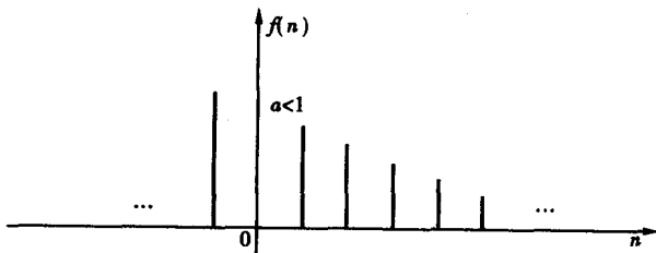
(c) 在实数 a < 1 时的实指数序列
