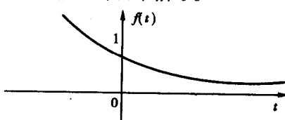
(b) f_2(t) = e^{-2t}
