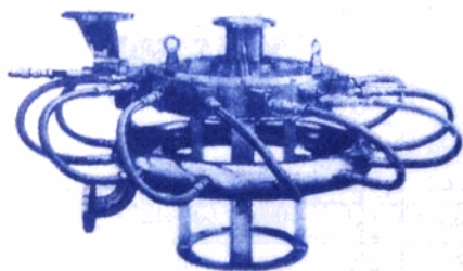
STJ 型扁平式超音速气流粉碎机
