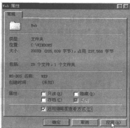
◎“属性”对话框
