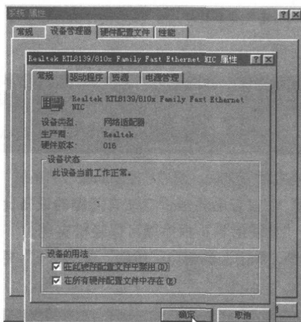
◎“常规”选项卡
