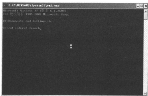
◎控制台模式
