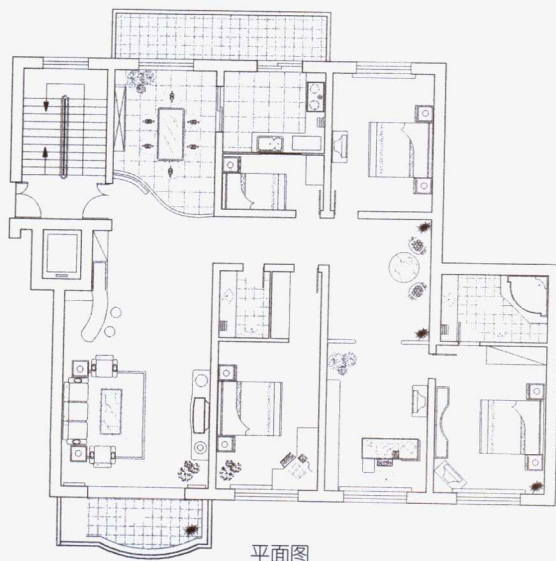
平面图
