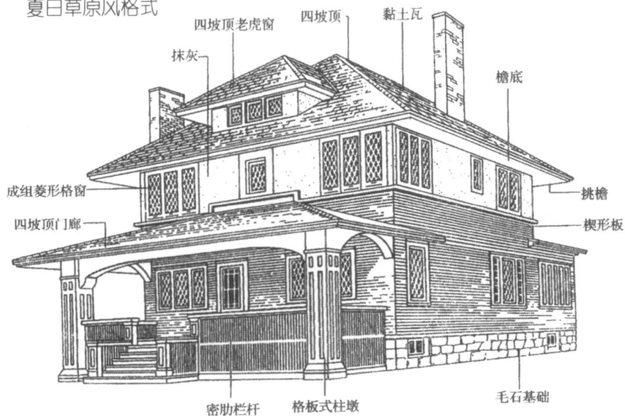
夏日草原风格式
