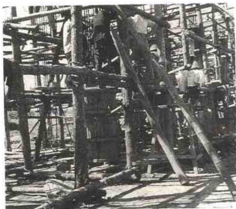
1965年裴河闸建设工地
