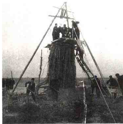
打扒坑井
