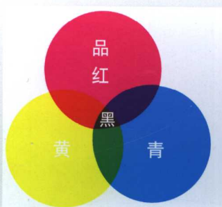
彩色图片 2 光的三补色
