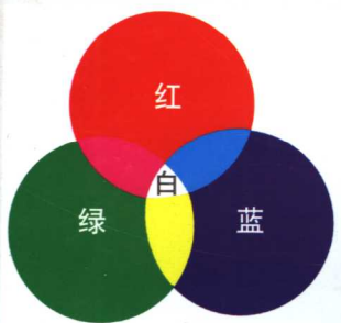
彩色图片 1 光的三原色
