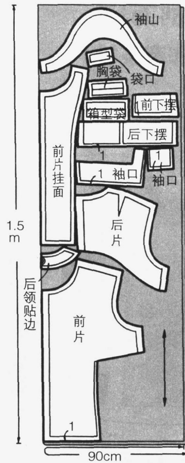
粘合衬裁剪图
